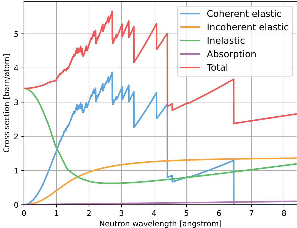
MgD2_sg136_MagnesiumDeuteride.ncmat
