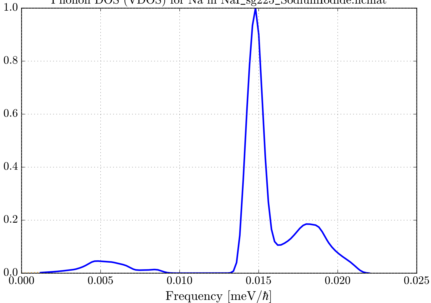
Phonon DOS (VDOS) for Na in NaI_sg225_SodiumIodide.ncmat
