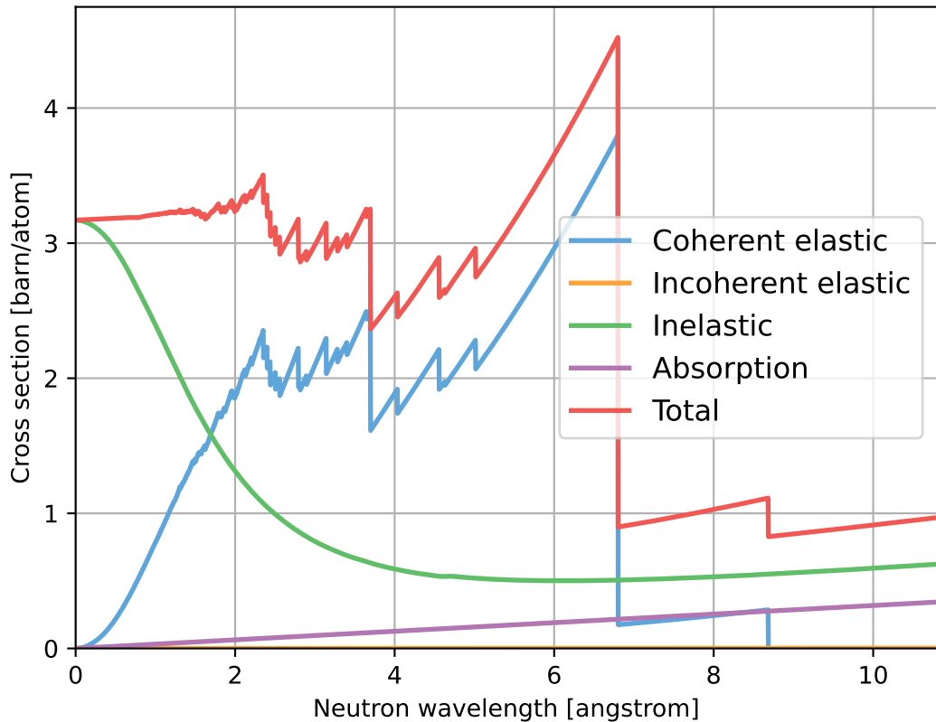
SiO2-beta_sg180_BetaQuartz.ncmat
