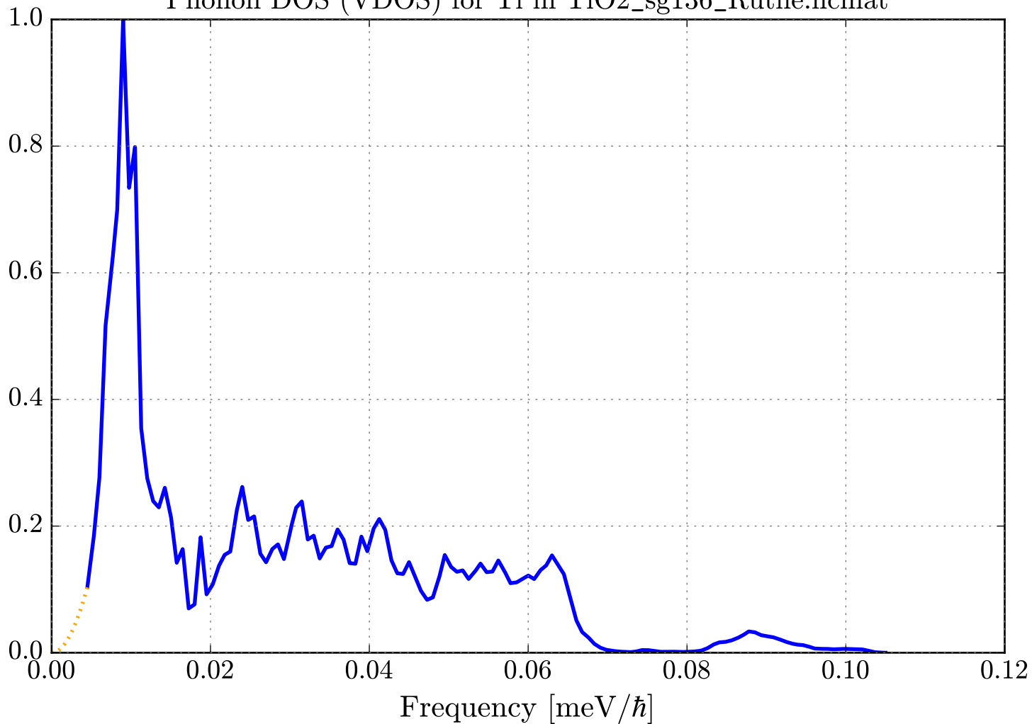
Phonon DOS (VDOS) for Ti in TiO2_sg136_Rutile.ncmat
