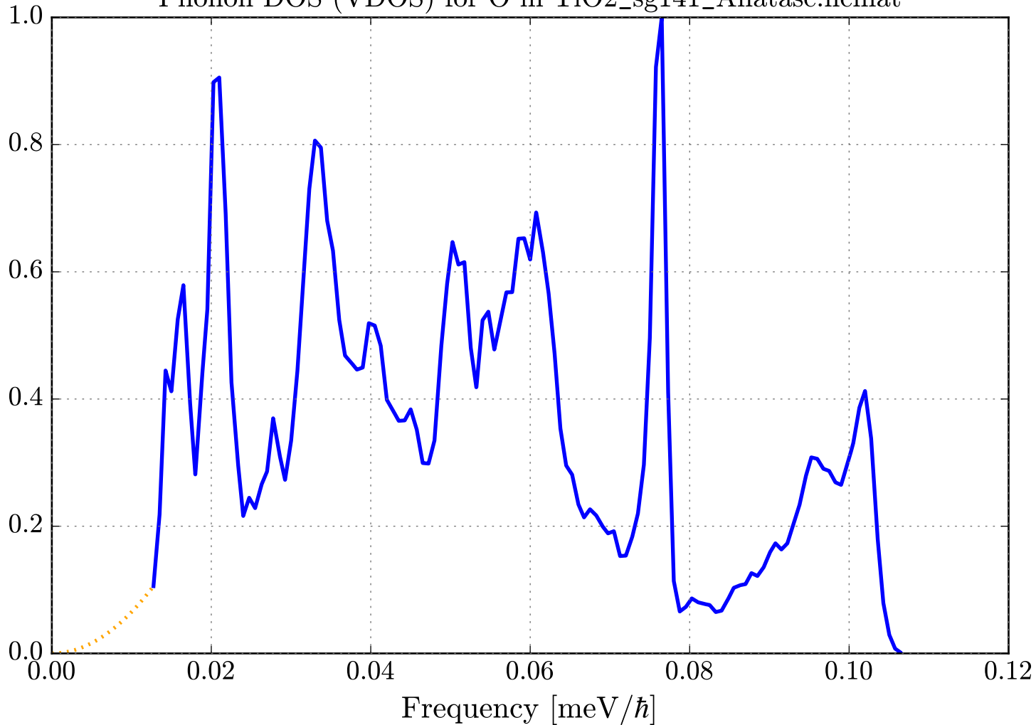
Phonon DOS (VDOS) for O in TiO2_sg141_Anatase.ncmat
