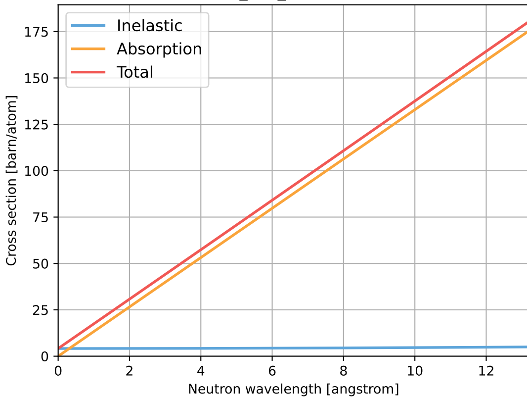
Xe_Gas_STP.ncmat
